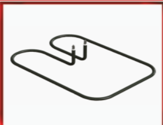
ТЭН В2-216/280-7,5/8,5/3,4Т220_000.185/1 Нержавик
